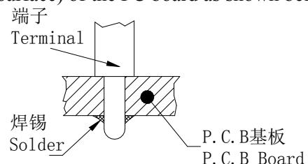
插脚式机种焊线图
